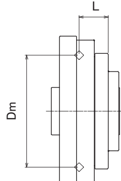
WPU-□-□-SDH
