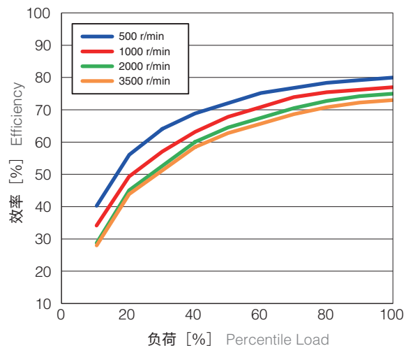
WPU-42-120
